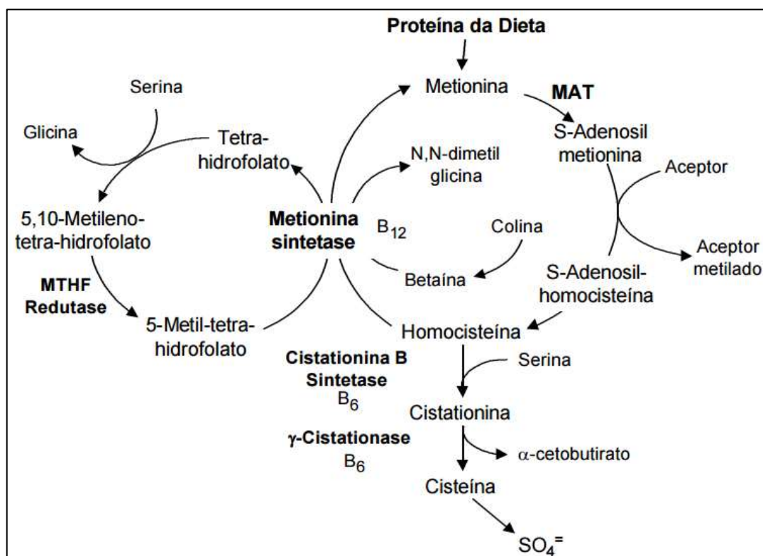
Figura 1. Vias metabólicas da Homocisteína.
